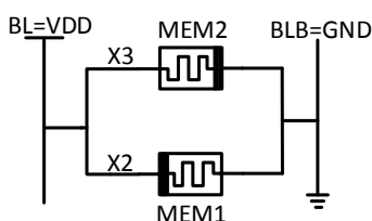
شکل (۲): مدار معادل نوشتن 0 در سلول پیشنهادی Figure (2): Equivalent circuit of writing 0 in the proposed cell.
