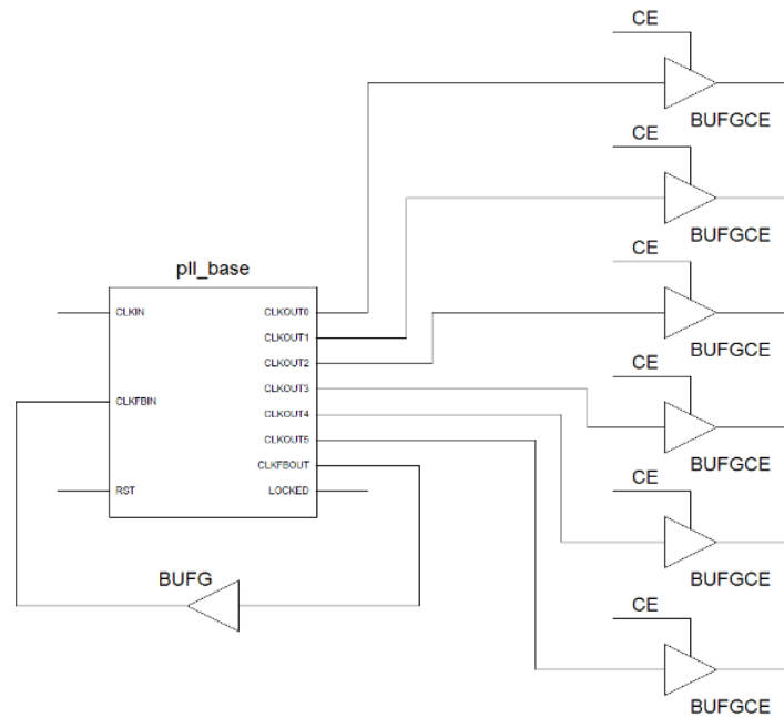
شکل (۳): نحوه به کارگیری بافر BUFVCE در ساختار اندازه‌گیر پهنای پالس Figure (3): How to use the BUFVCE buffer in the structure of pulse measurement
