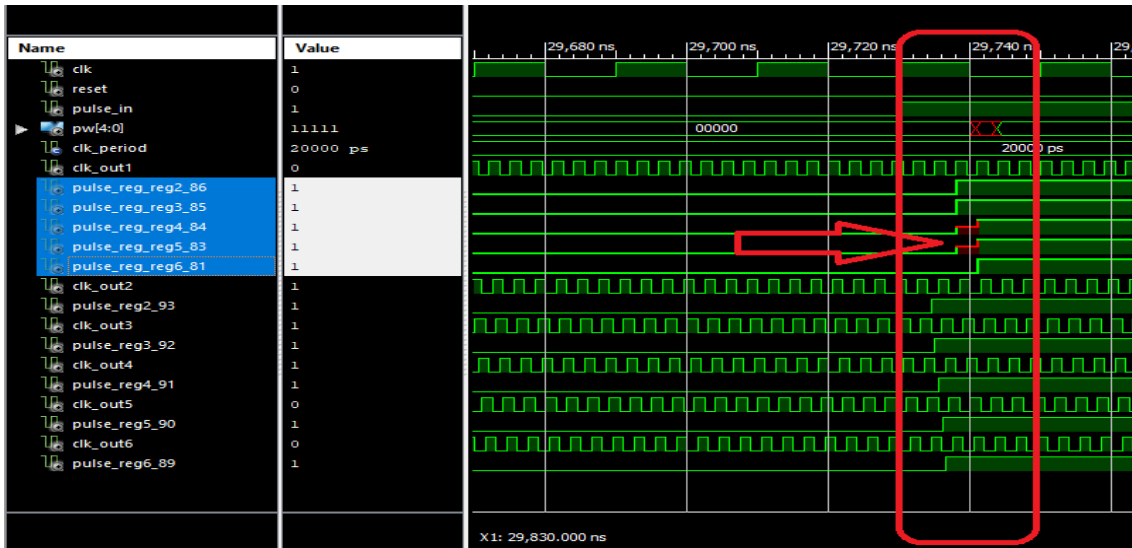
شکل (۶): تأخیر اجتناب‌ناپذیر در معماری کلی-دقیق برای انتقال داده Figure (6): Inevitable delays in coarse-fine architecture for data transfer
