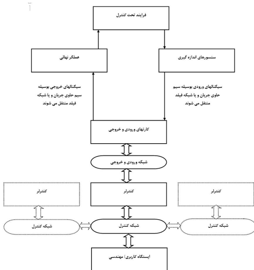
شکل (۲): ساختار عملکردی سیستم کنترل Figure (2): Control system functional structure
