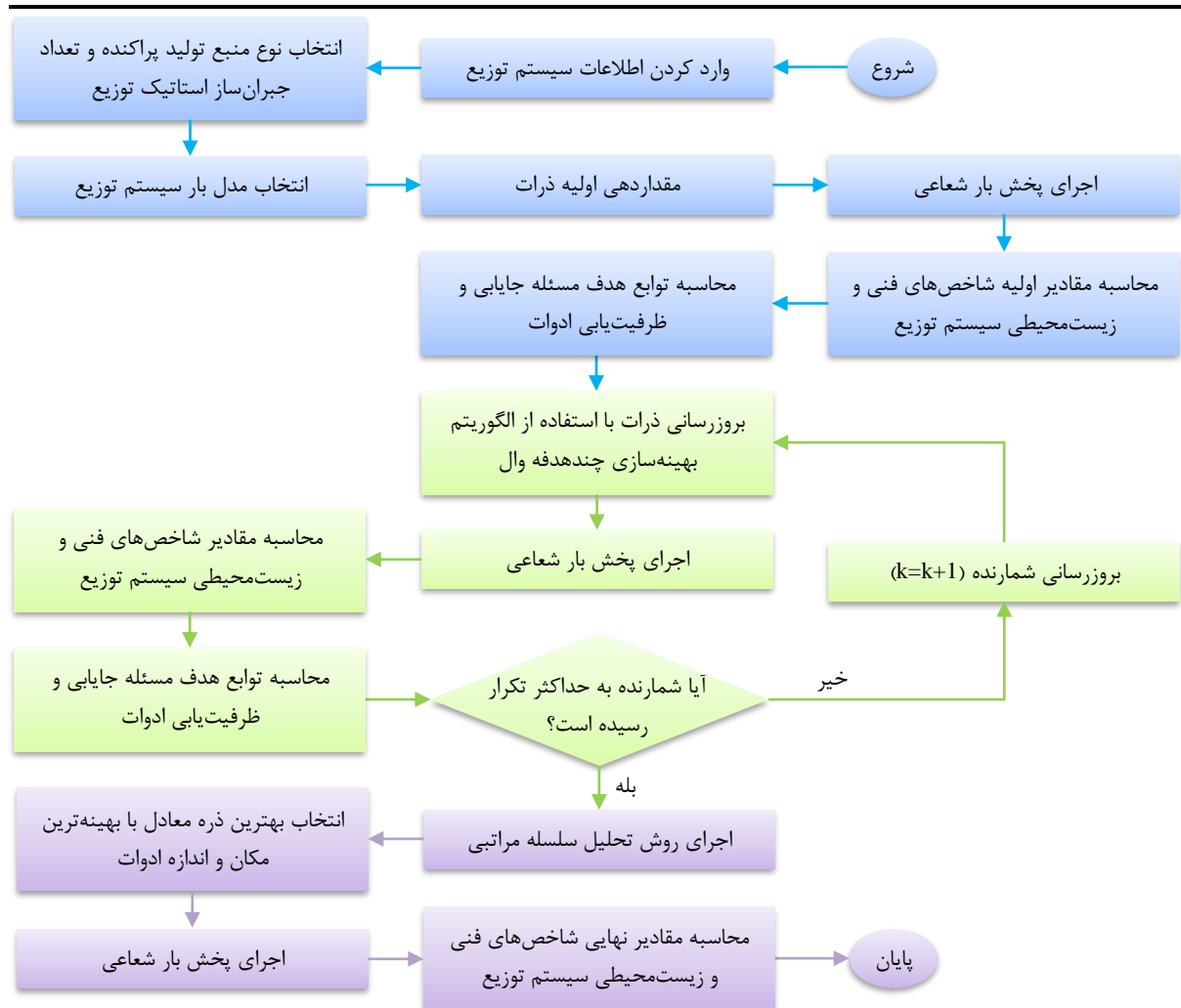
شکل (۲): فلوچارت روش پیشنهادی برای بهینه‌سازی چندهدفه مکان و اندازه انواع منابع تولید پراکنده و جبران‌ساز استاتیک توزیع Figure (2): Flowchart of the proposed method for multi-objective optimizing the location and size of DGs and DSTATCOM
