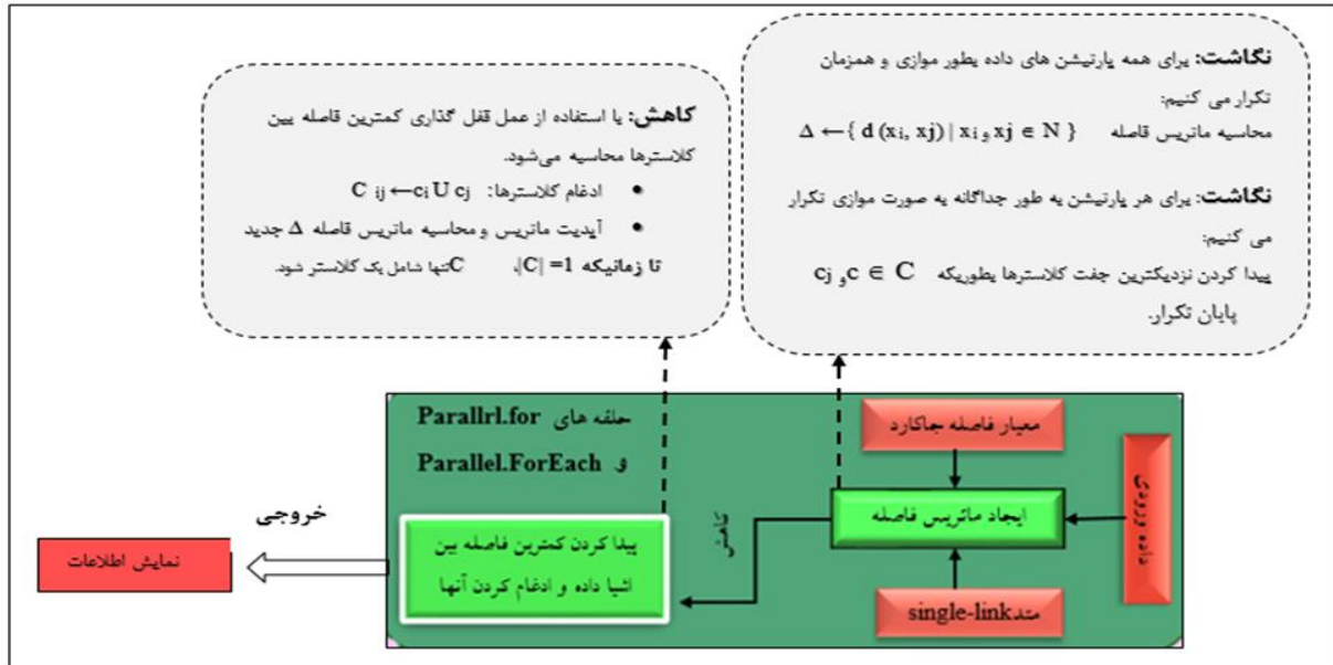
شکل (۲): چارچوب ارائه‌شده برای پیاده‌سازی الگوریتم خوشه‌بندی سلسله‌مراتبی متراکم بر اساس روش نگاشت-کاهش Figure (2): The presented framework to map-reduce implementation of agglomerative hierarchical clustering
