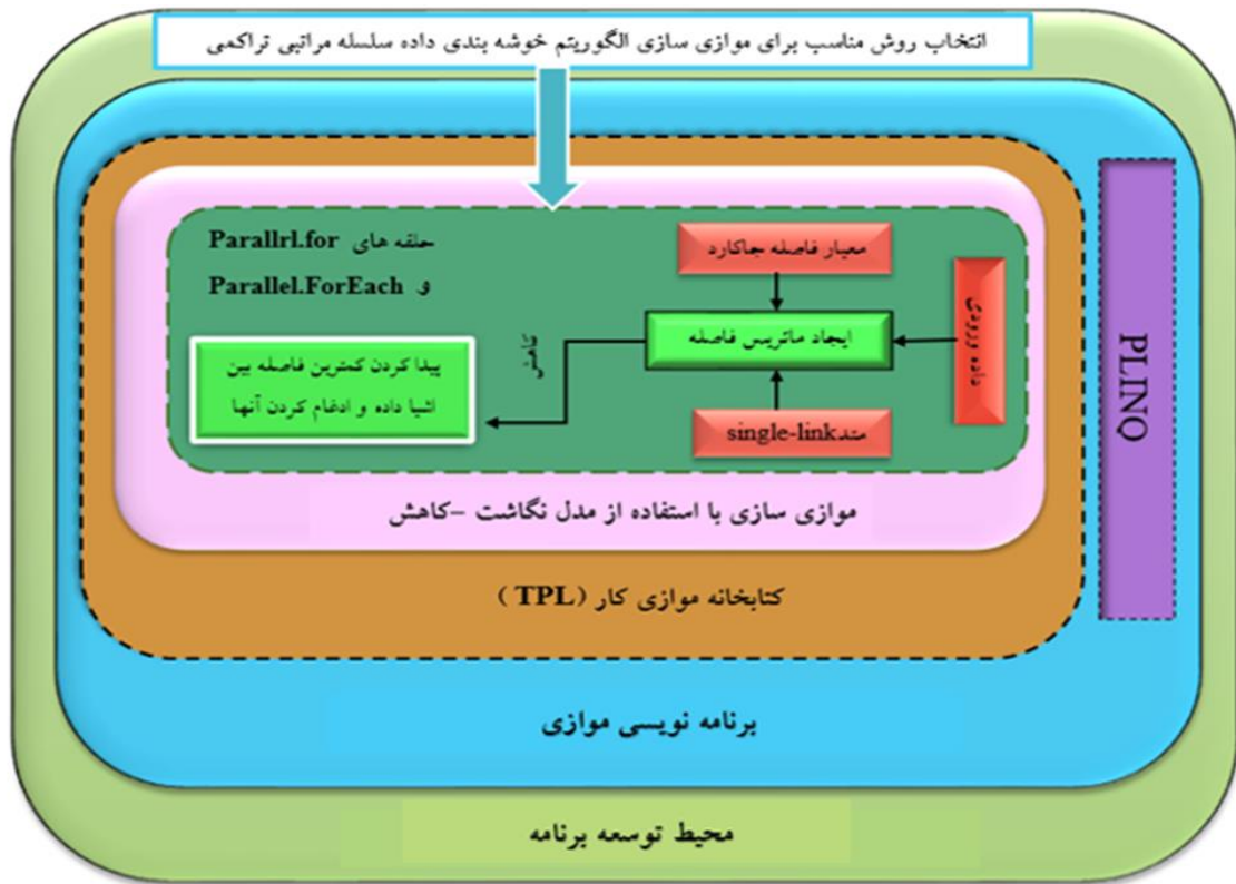
شکل (۴): مراحل توسعه الگوریتم ترتیبی خوشه‌بندی سلسله‌مراتبی تراکمی به صورت موازی Figure (4): Developing steps of the parallel agglomerative hierarchical clustering algorithm
