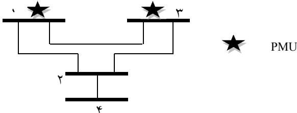
شکل (۲): میزان افزونگی سیستم ۴- باس Fig (2): Measurement redundancy in 4-bus system
