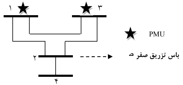
شکل (۳): تأثیر گره تزریق صفر روی رویت‌پذیری باس‌ها Fig. (3): Impact of zero injection bus on observability
